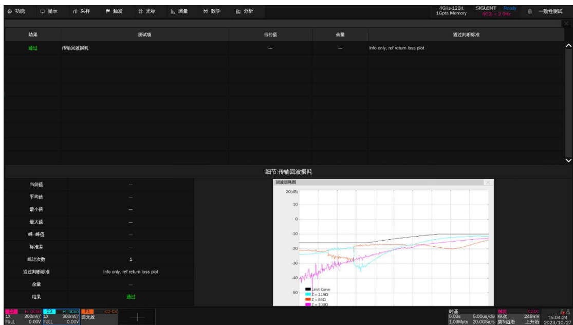
图 6-19 发送器回波损耗测试结果参考
