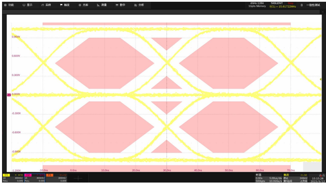
图 6-3 模板测试的波形展开细节
