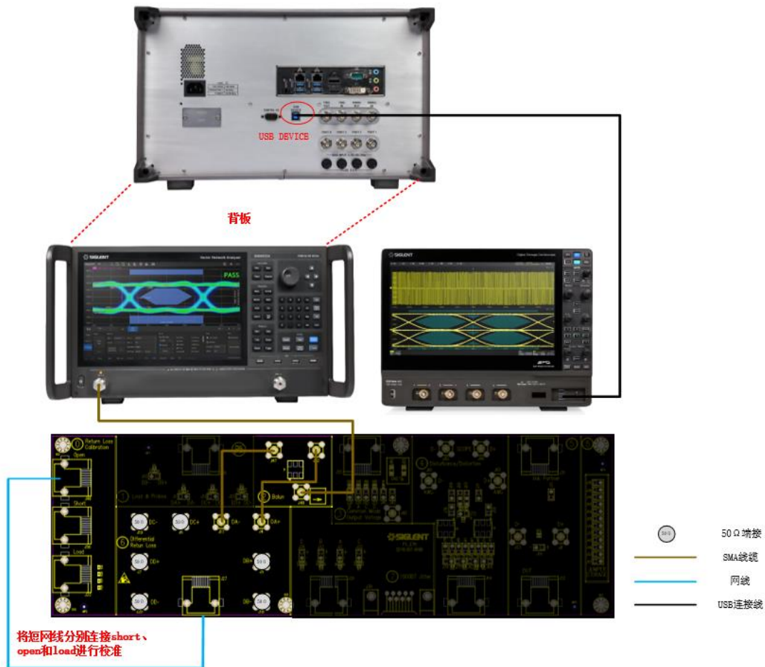
图 6-17 VNA 校准环境
