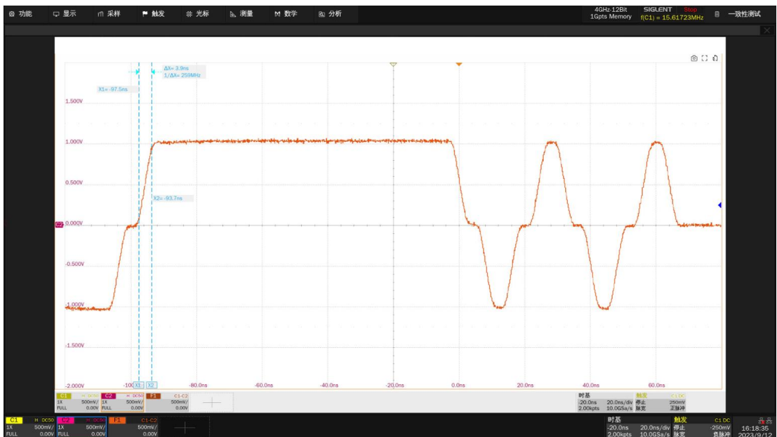
图 6-11 上升时间测试波形的展开细节
