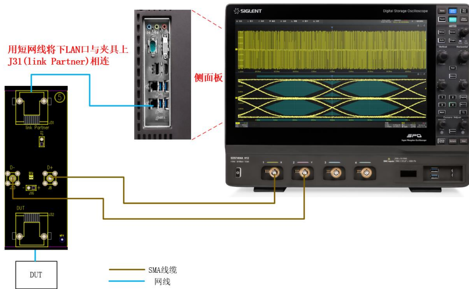
图 5-5 SDS7000A 为 Link Partner 下的 SMA 线缆连接
