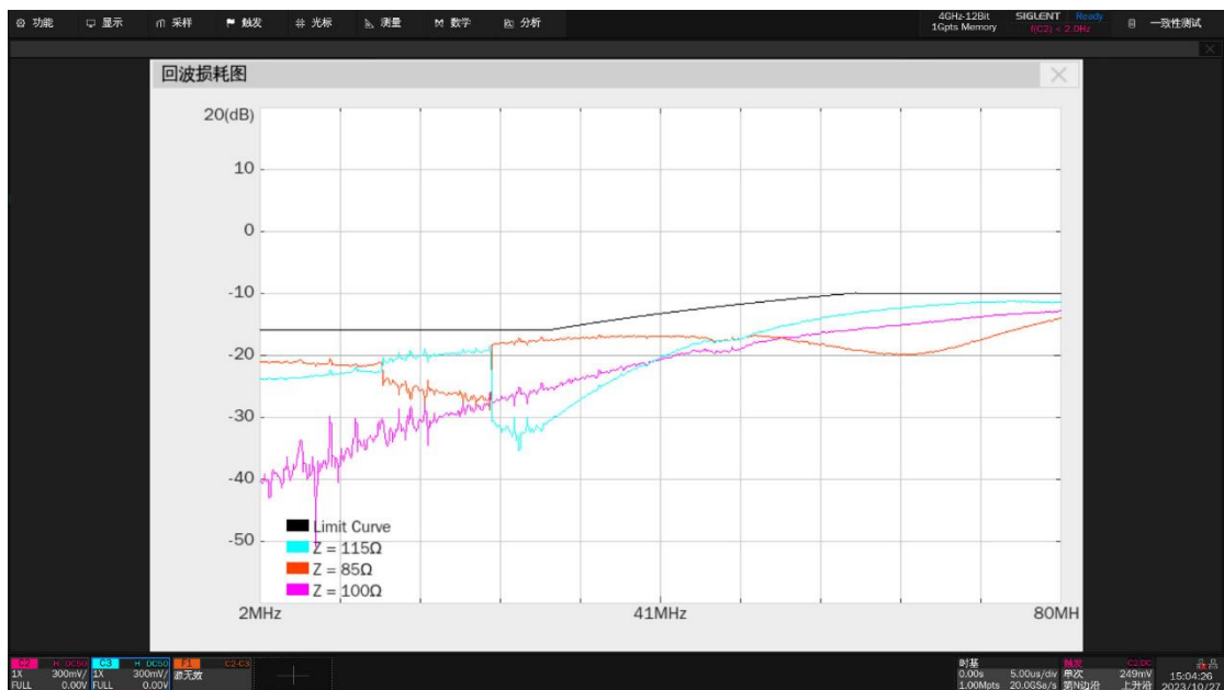
图 6-20 发送器回波损耗波形细节
