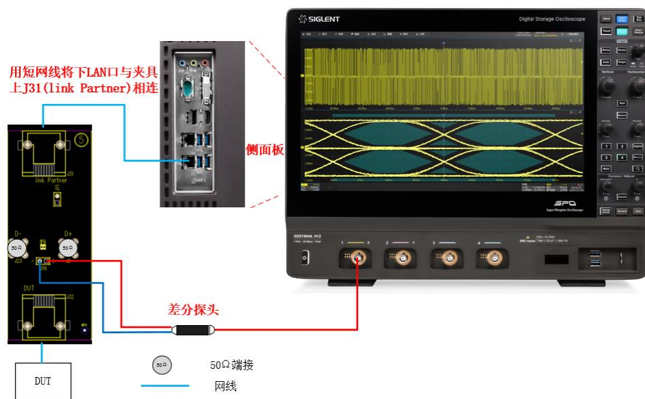
图 5-6 SDS7000A 为 Link Partner 下的有源差分探头连接
