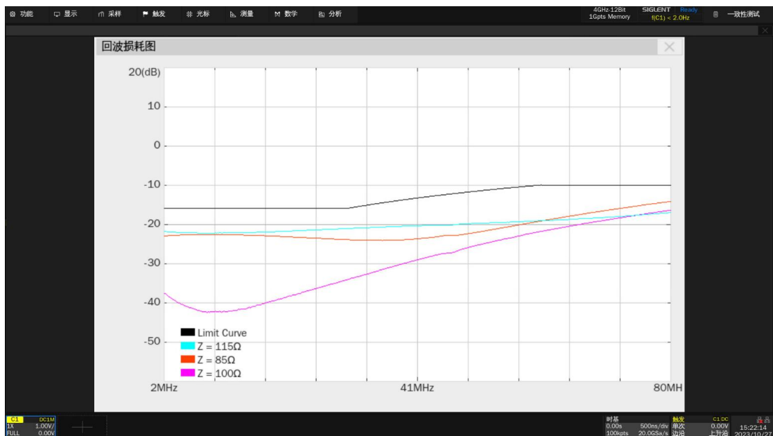
图 6-24 接收器回波损耗波形细节
