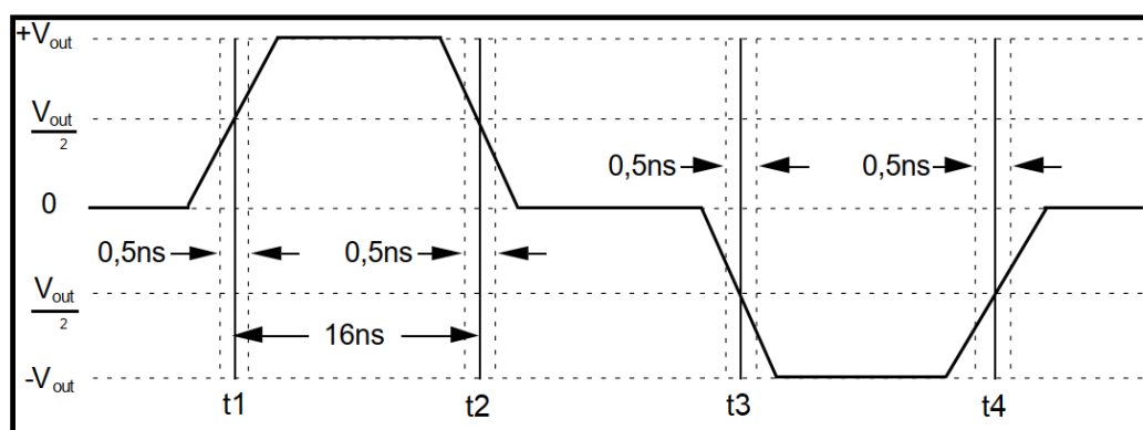
图 6-12 占空比失真测试
